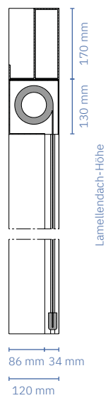
Schnittansicht A-A
