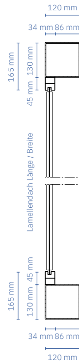
Schnittansicht B-B
